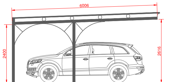
VISTA LATERALE
